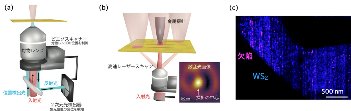
図 3 (a)集光位置のリアルタイム補正機構。反射光から得られた対物レンズの位置ずれ情報を元にピエゾスキャナーにフィードバック信号を送る。(b)探針と入射光の相対位置補正機構。散乱光画像内の輝点から探針の中心位置を検出する。(c) 広視野・長時間・超解像ラマンイメージングによる二次元材料 ( \text{WS}_2 ) の表面構造解析。 \text{WS}_2 と欠陥それぞれに由来するラマン散乱信号強度で画像化。
