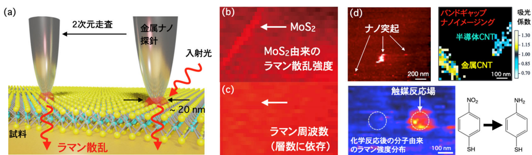
図 2 TERS によるナノ分子構造・物性解析に関する研究の概要。(a) TERS の概要図。(b)、(c)MoS 2 由来のラマン散乱光の強度と周波数で画像化した MoS 2 表面 (d) TERS を用いたナノ物性解析例 (二次元材料上のナノサイズの突起構造、カーボンナノチューブ (CNT) のナノ吸光係数イメージング、金属触媒の反応特性の可視化)。
